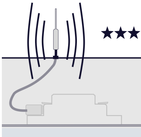
Figuur 2: Het verdikte gedeelte van antenne geheel door de metalen behuizing/schakelkast naar buiten leiden plus 1,5cm van de antennekabel
