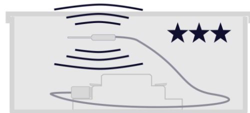
Figuur 10: Plaats de antenne vrij in een kunststof kabeldoos/behuizing (niet tegen kunststof aan)
